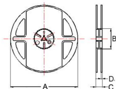
Reel Dimensions
